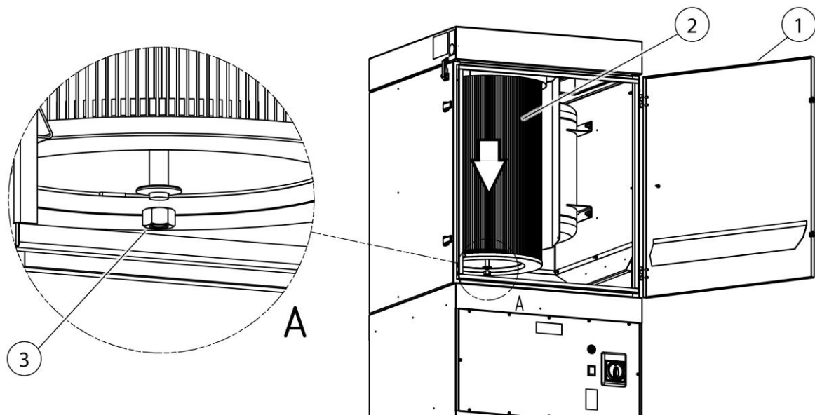
Abb. 9: Filterwechsel
