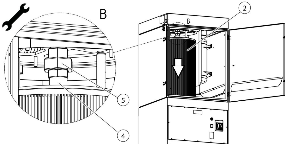
Abb. 10: Filterpatrone entnehmen
