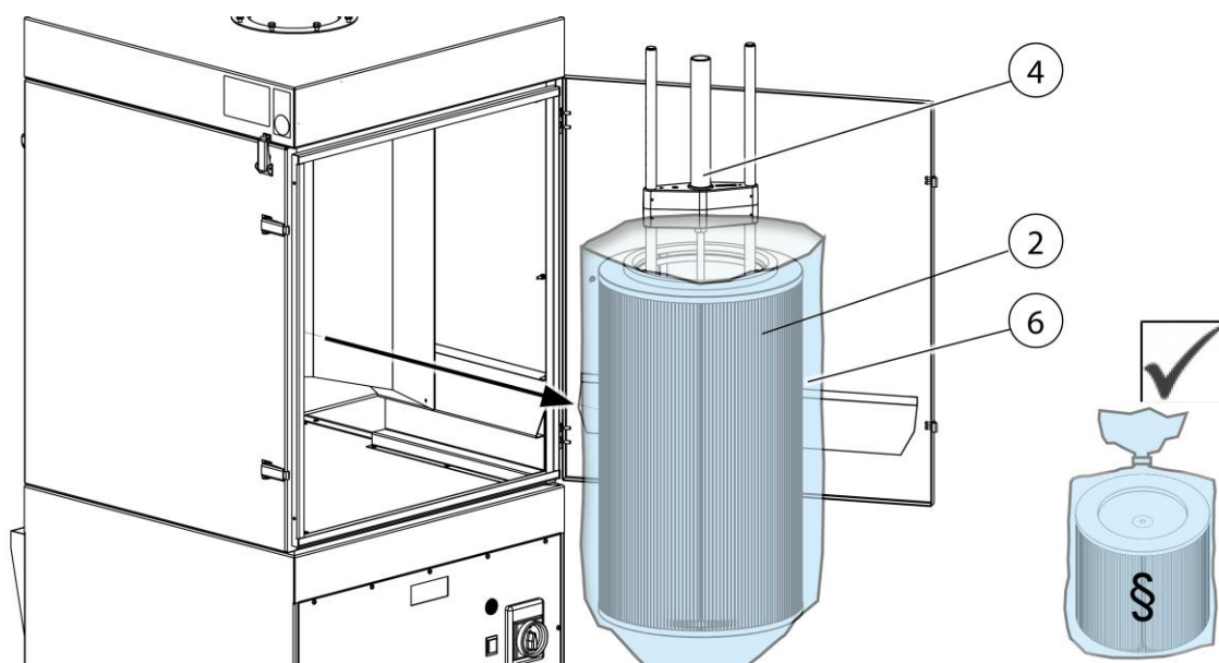
Abb. 11: Filterpatrone Entnehmen
