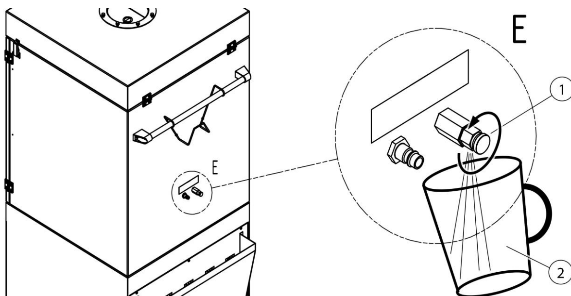
Abb. 8: Kondensat ablassen
