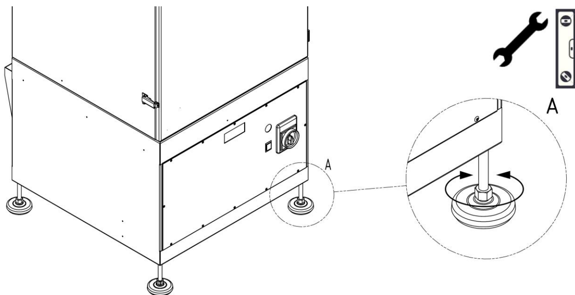
Abb. 2: Produkt ausrichten
